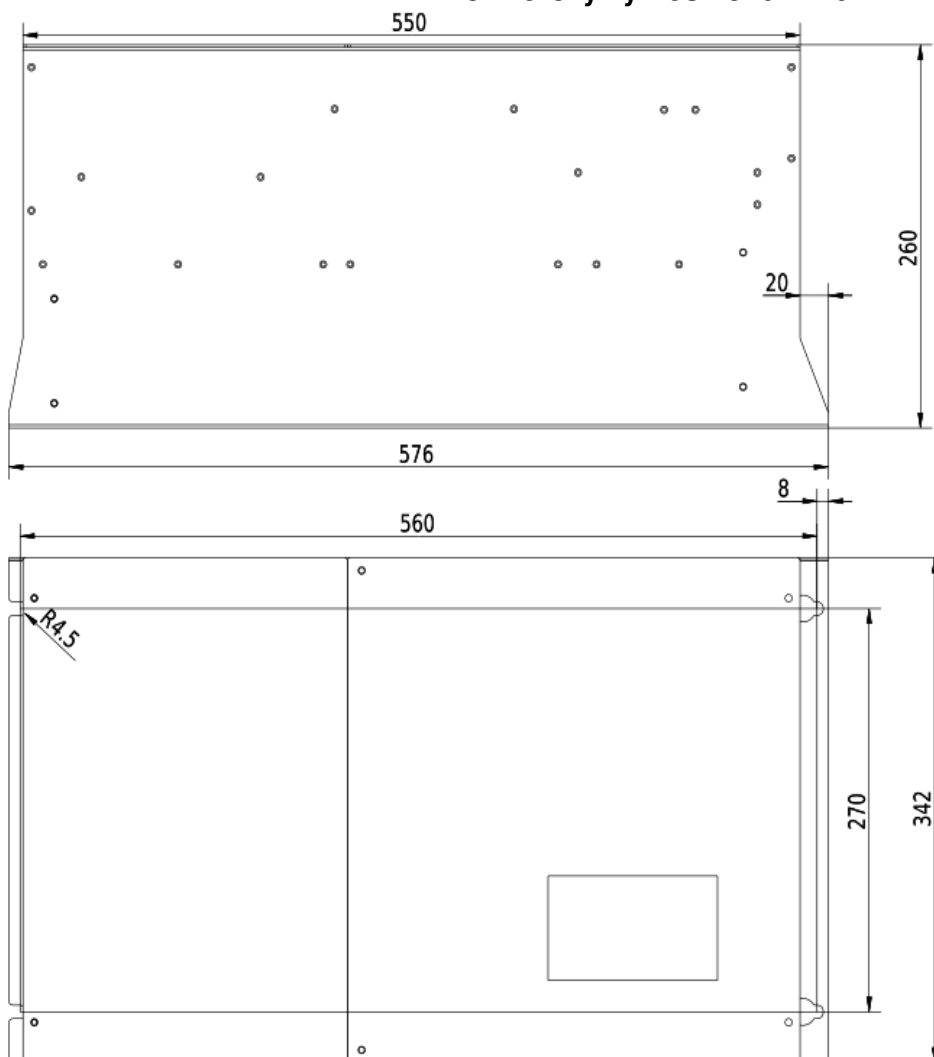
Rozmerový výkres V8 10 - 110kW 4 T1100
