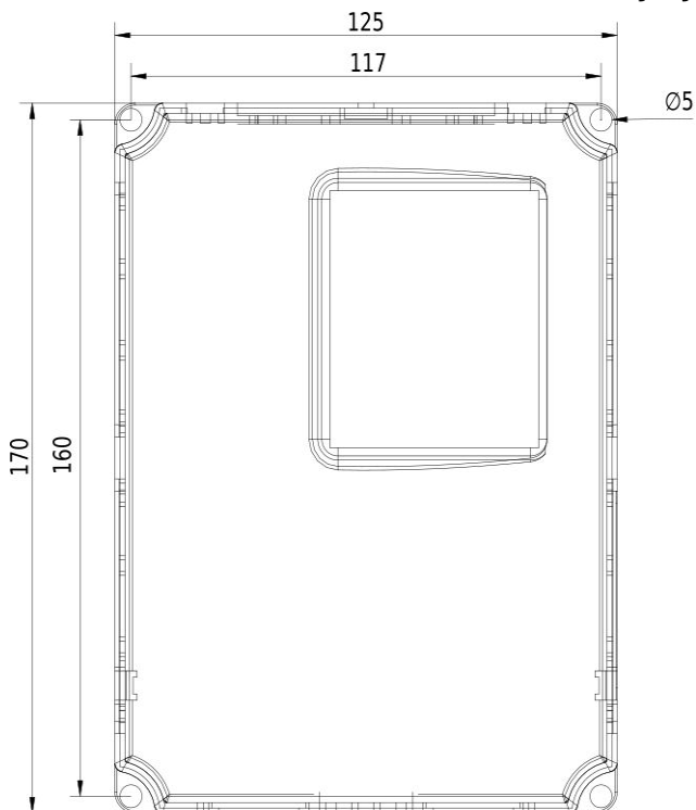
Rozmerový výkres V810 - 2,2kW 2S0022
