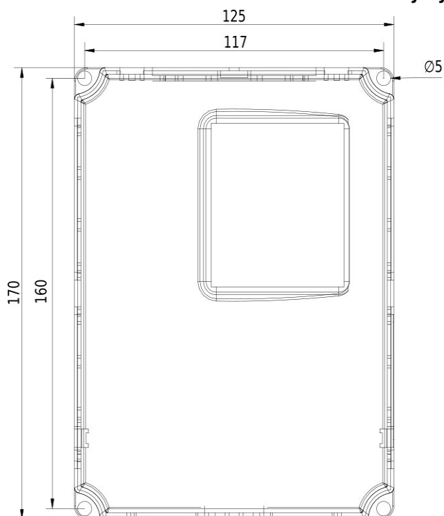
Rozmerový výkres V8 10 - 1,5kW 2S0015
