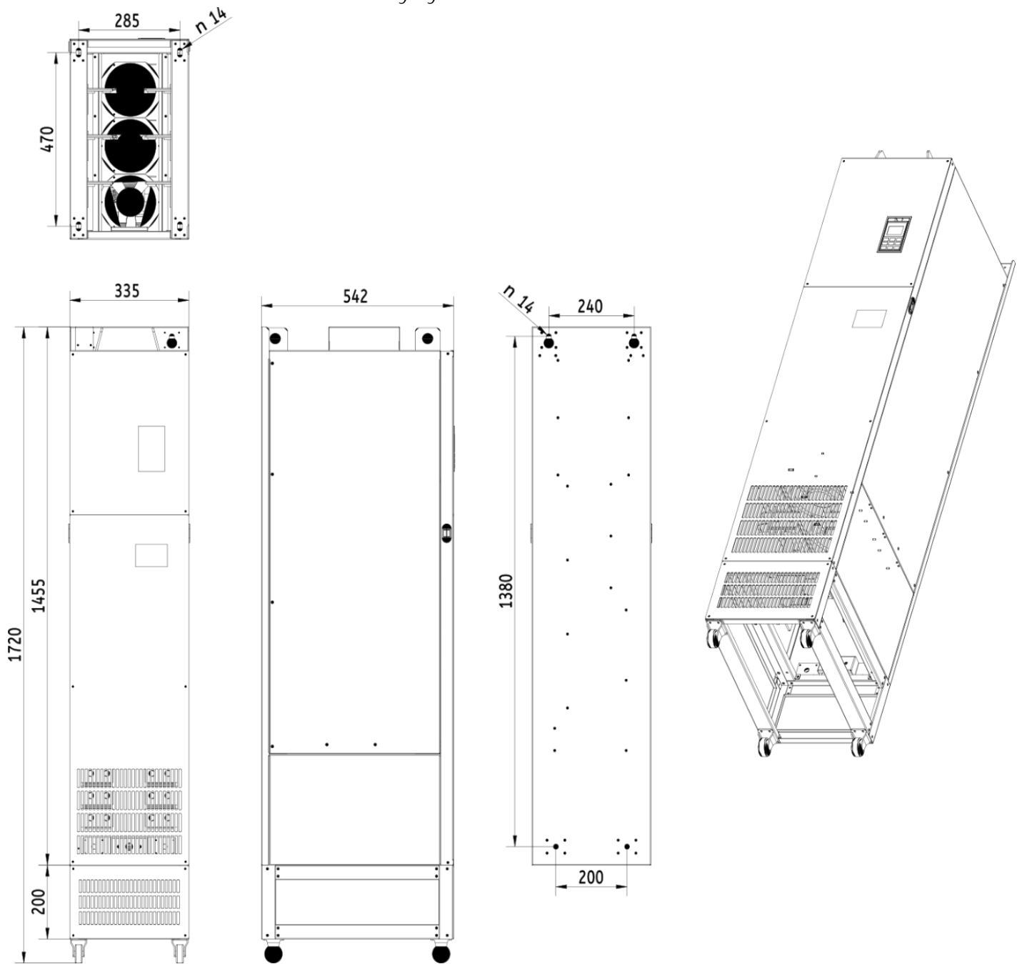
Rozmerový výkres V900 - 400kW 4T4000
