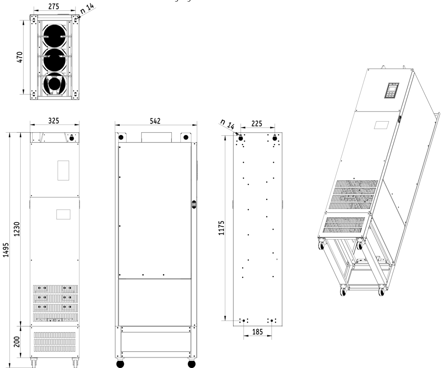
Rozmerový výkres V900 - 315kW 4T3150
