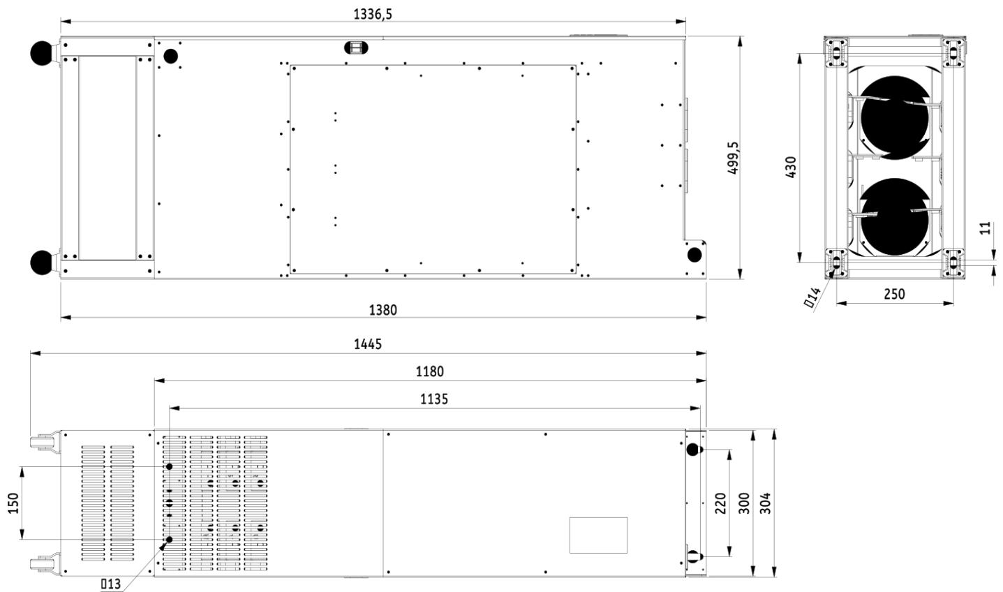
Rozmerový výkres V900 - 250kW 4T2500
