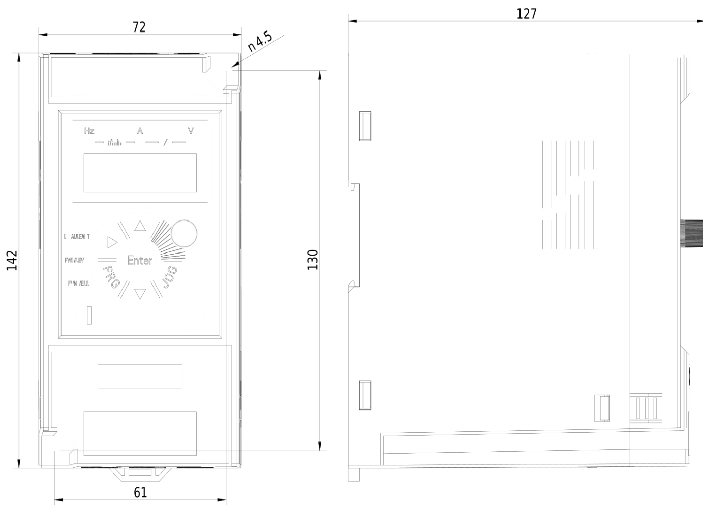
Rozmerový výkres V900 - 0,75kW 4T0007
