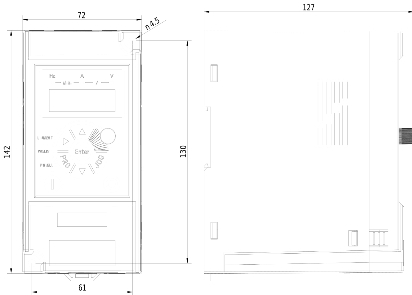
Rozmerový výkres V900 - 0,75kW 2S0007
