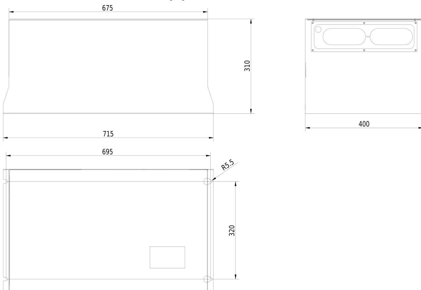
Rozmerový výkres V900 - 160kW 4T1600
