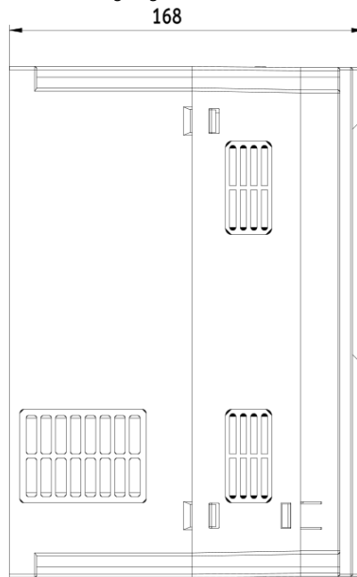
Rozmerový výkres V900 - 15kW 4T0150
