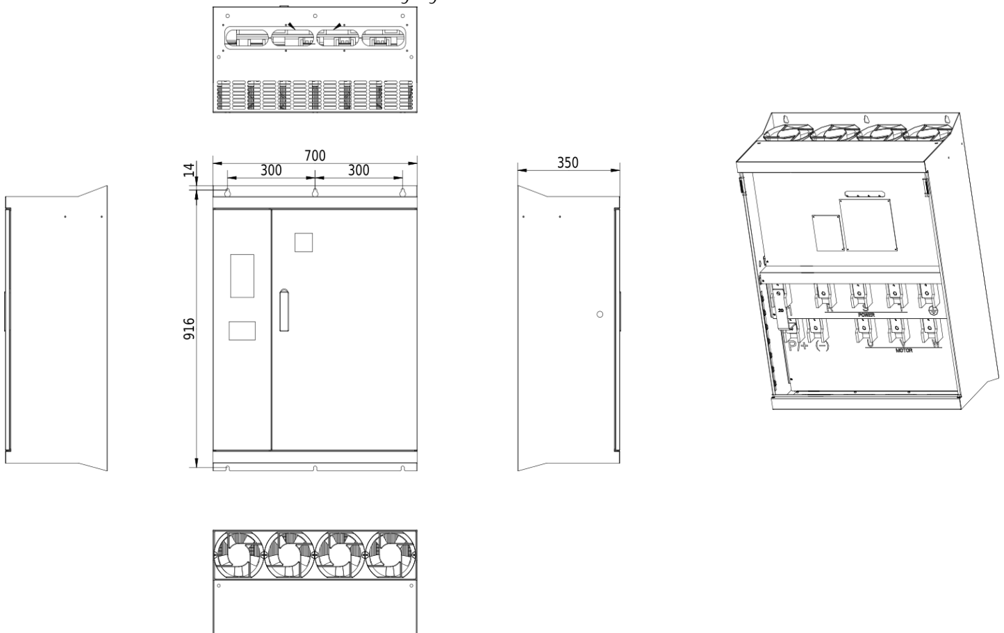
Rozmerový výkres V810 - 350kW 4T3500
