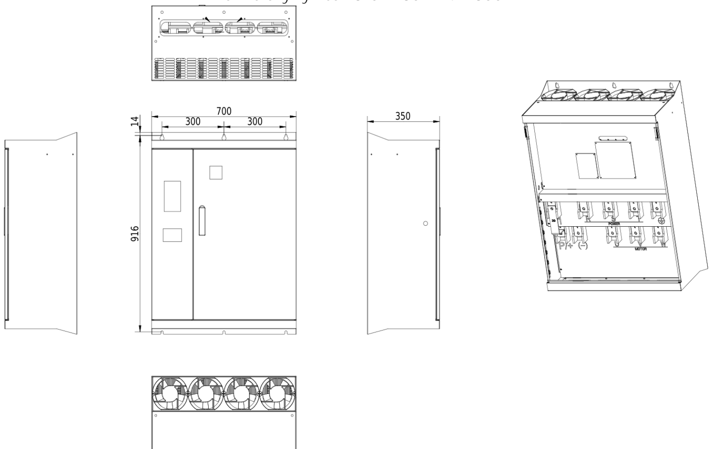
Rozmerový výkres V810 - 280kW 4T2800
