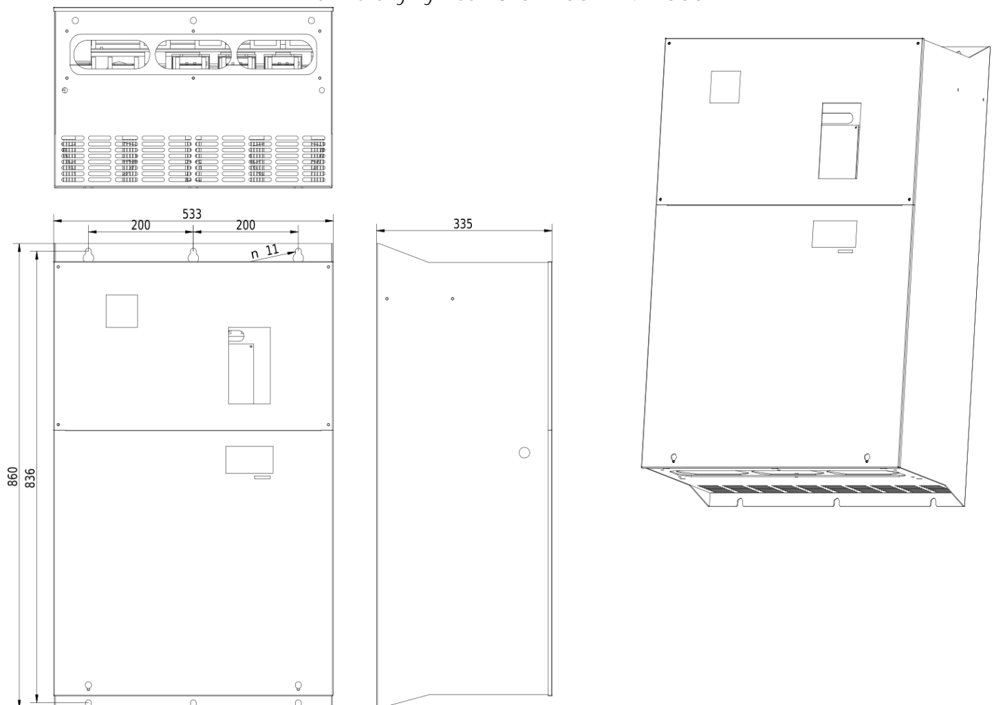
Rozmerový výkres V810 - 200kW 4T2000
