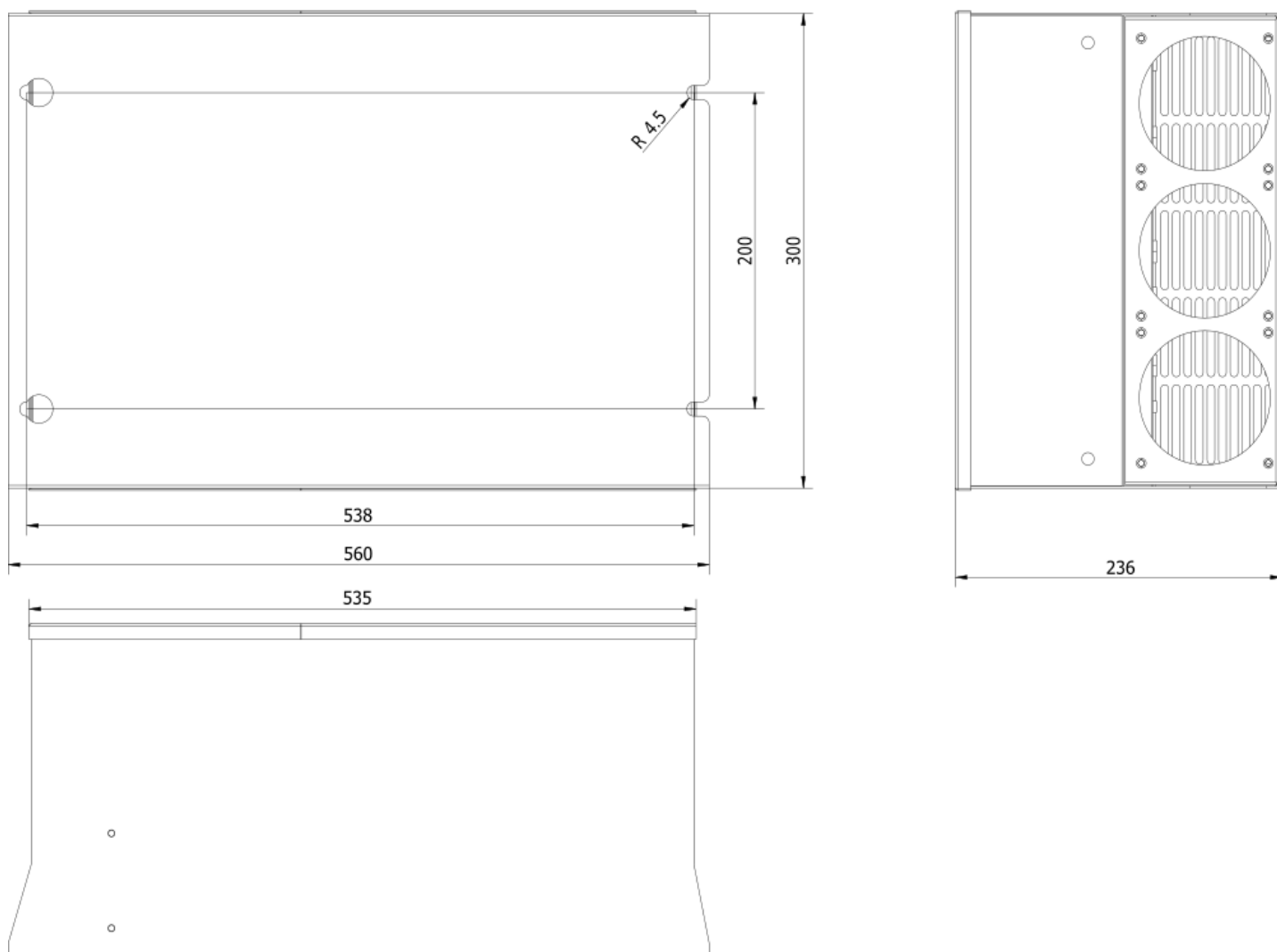
Rozmerový výkres V810 - 75kW 4T0750
