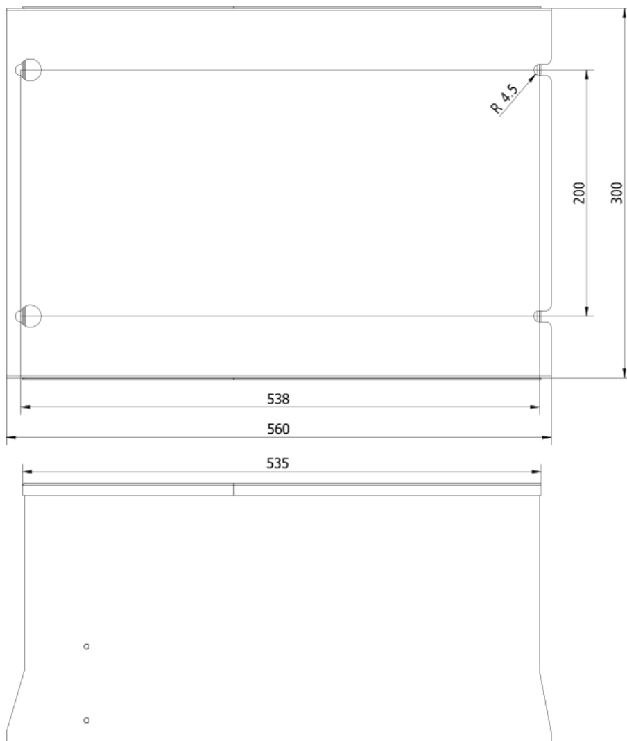
Rozmerový výkres V810 - 55kW 4T0550
