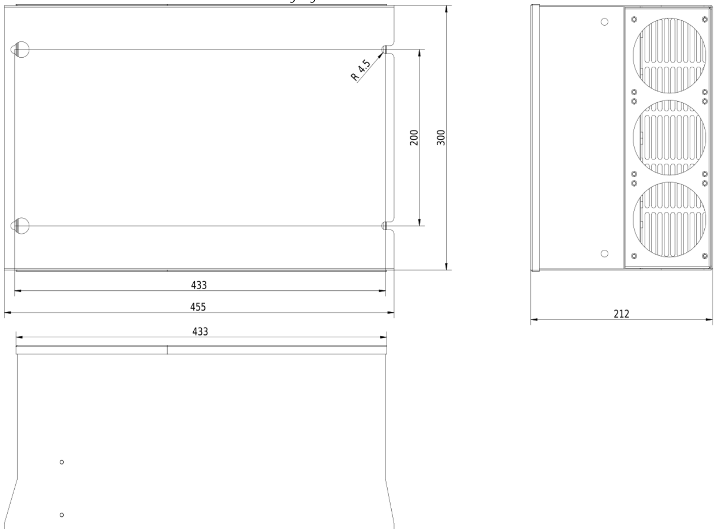
Rozmerový výkres V810 - 45kW 4T0450
