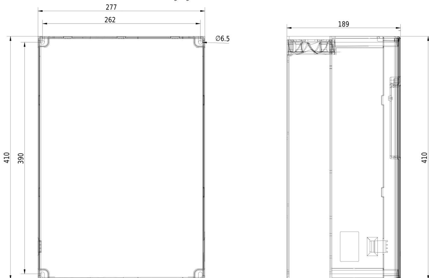
Rozmerový výkres V810 - 37kW 4T0370
