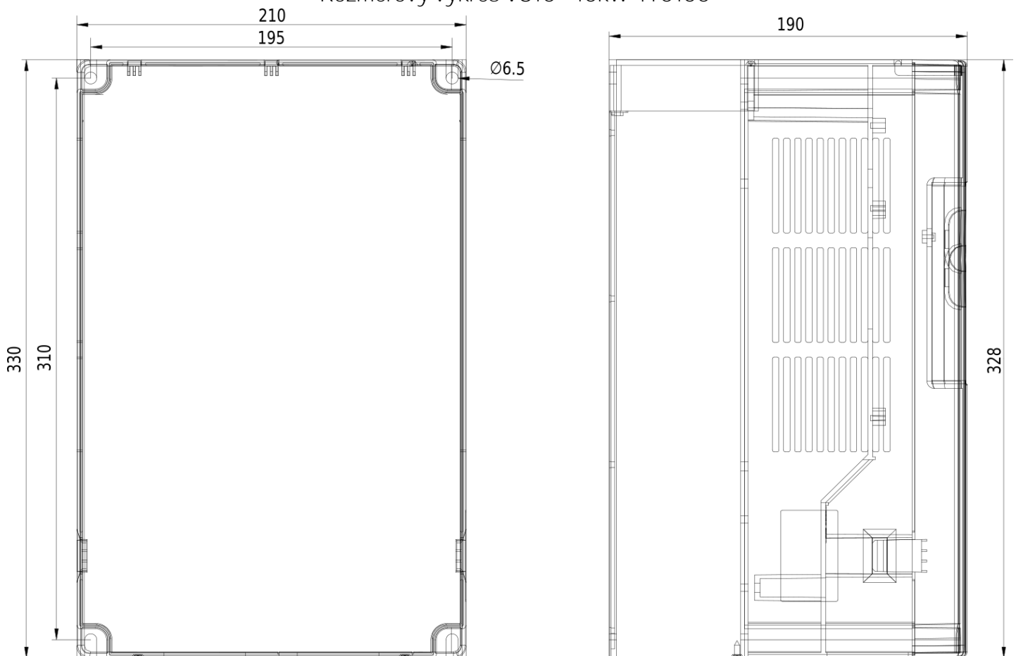
Rozmerový výkres V810 - 15kW 4T0150
