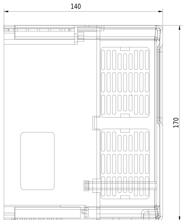
Rozmerový výkres V810 - 2,2kW 4T0022
