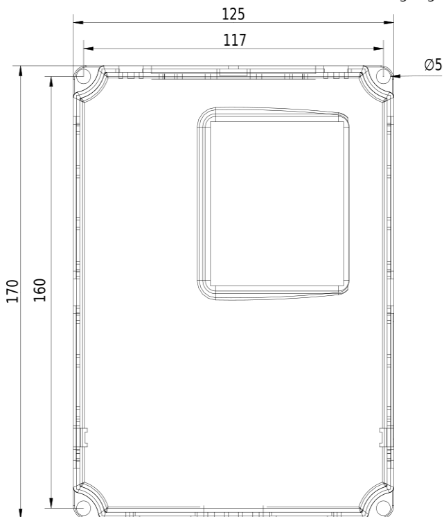
Rozmerový výkres V810 - 0,75kW 2S0007
