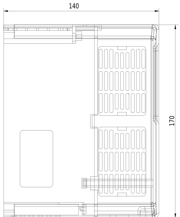
Rozmerový výkres V810 - 0,75kW 2S0007
