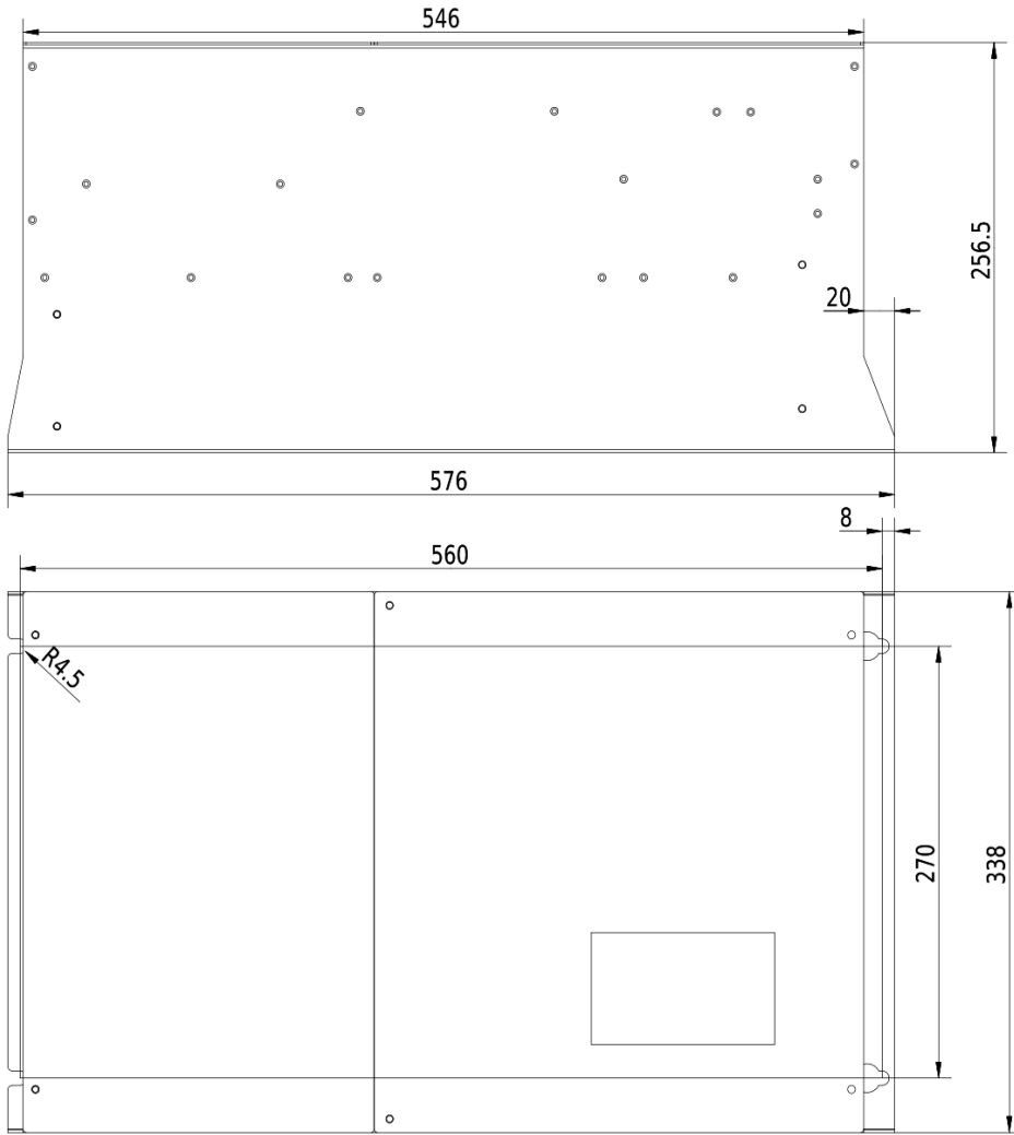
Rozmerový výkres V800 - 90kW 4T0900
