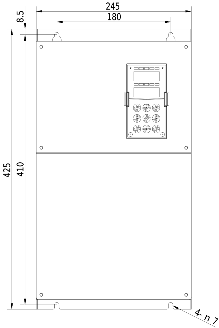
Rozmerový výkres V800 - 45kW 4T0450
