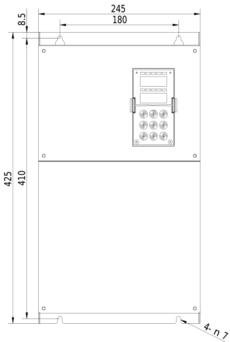
Rozmerový výkres V800 - 37kW 4T0370
