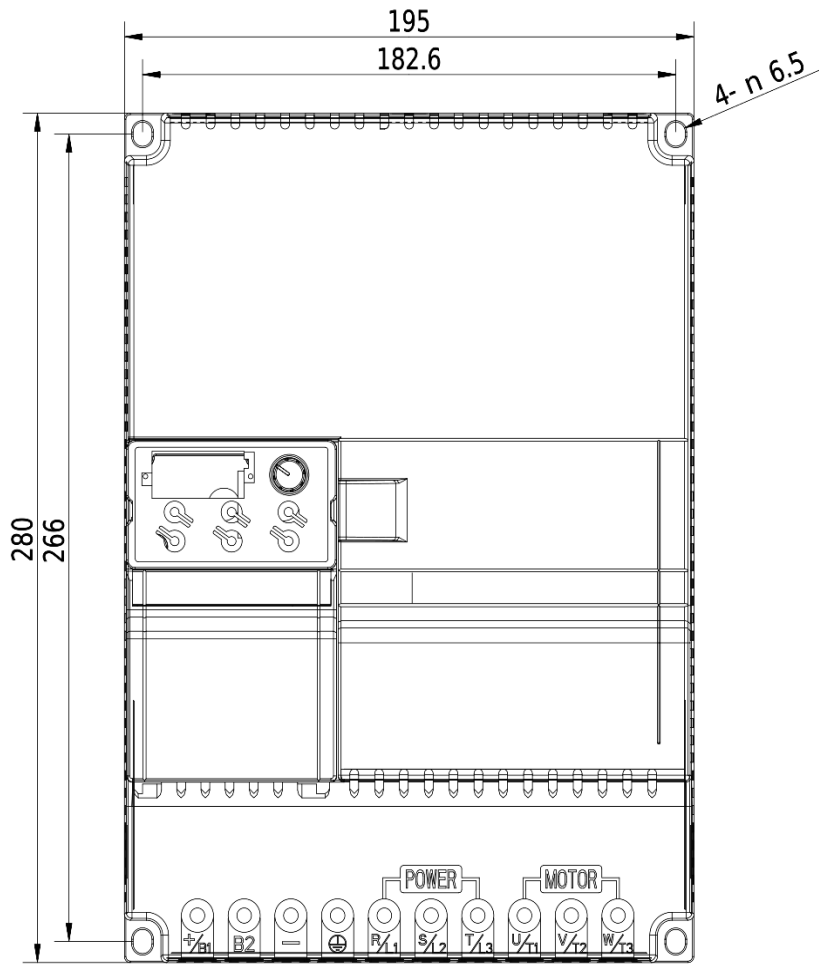
Rozmerový výkres V800 - 30kW 4T0300
