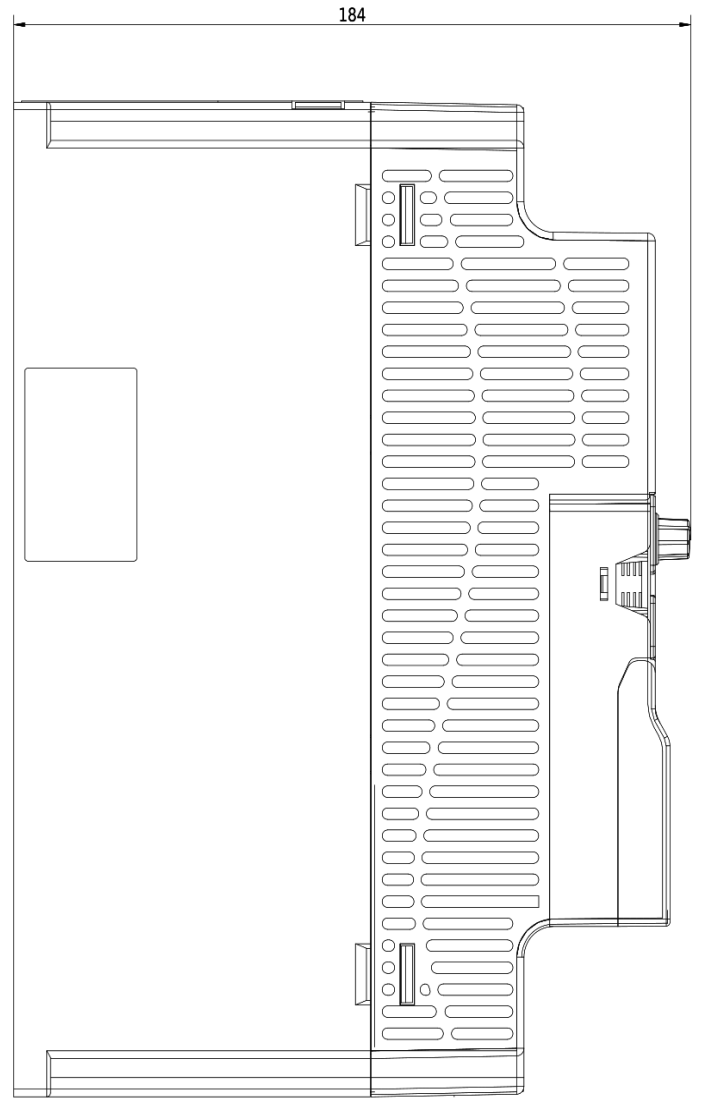
Rozmerový výkres V800 - 15kW 4T0150
