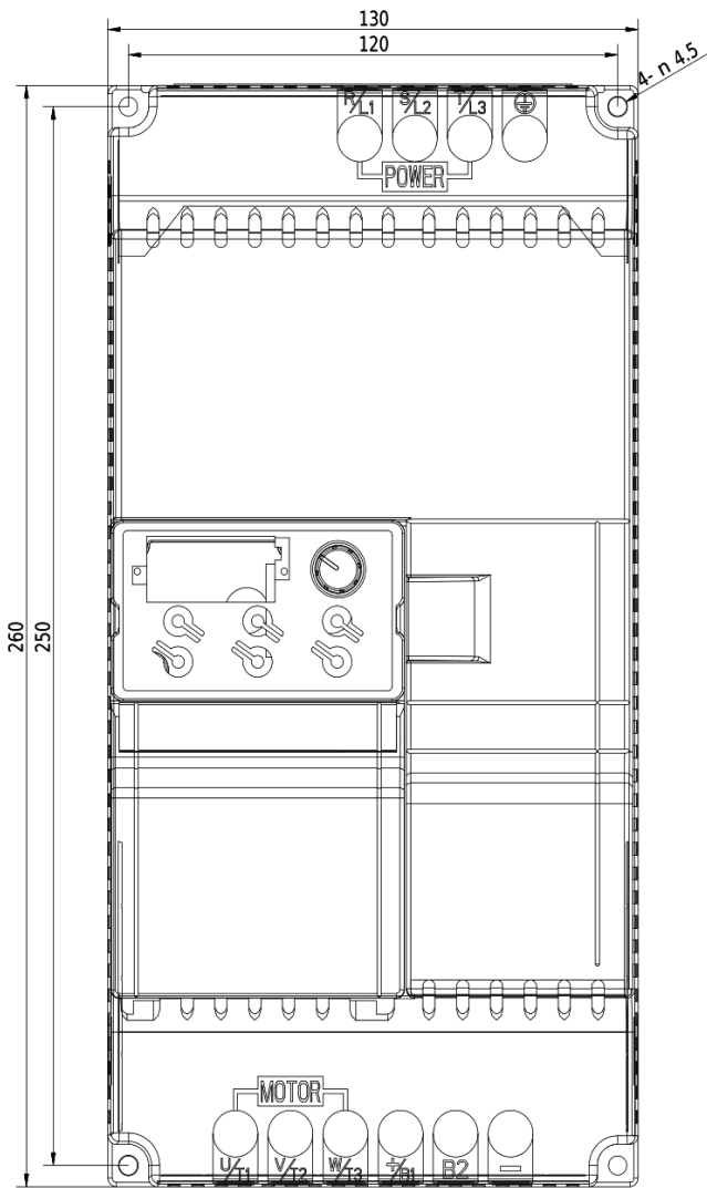
Rozmerový výkres V800 - 15kW 4T0150
