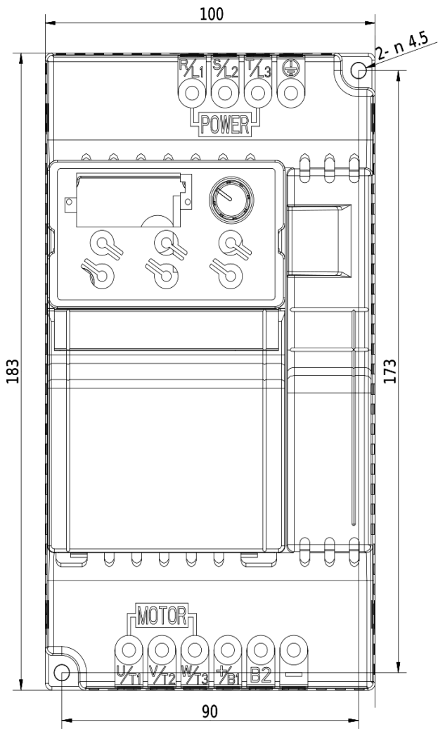
Rozmerový výkres V800 - 7,5kW 4T0075
