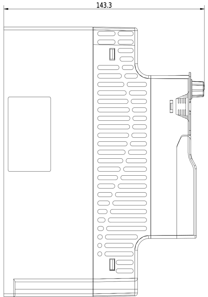
Rozmerový výkres V800 - 5,5kW 4T0055
