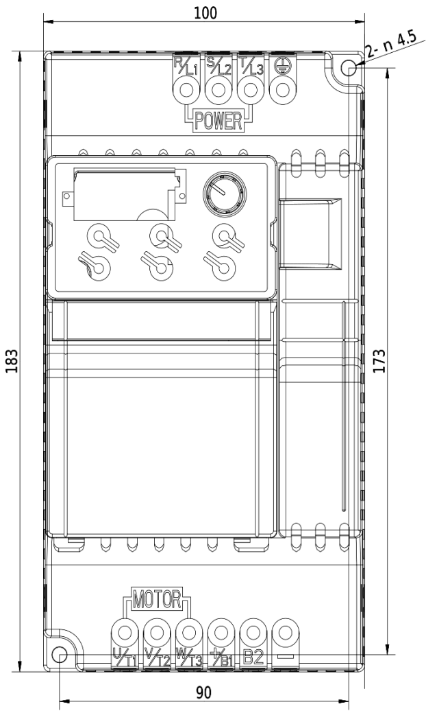
Rozmerový výkres V800 - 5,5kW 4T0055
