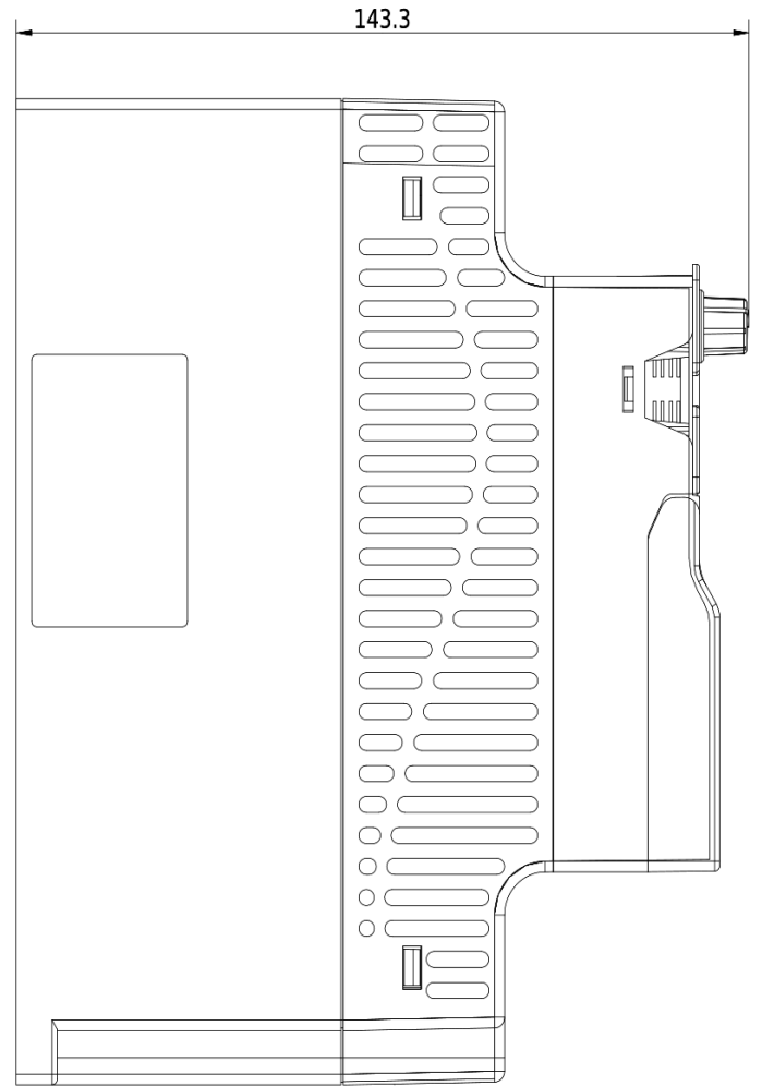
Rozmerový výkres V800 - 4kW 4T0040
