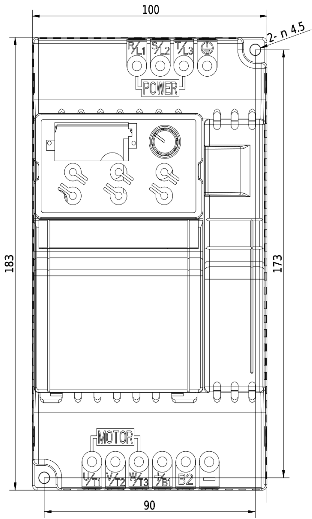
Rozmerový výkres V800 - 4kW 4T0040
