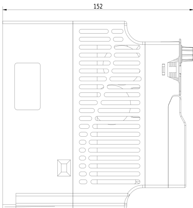
Rozmerový výkres V800 - 2,2kW 4T0022
