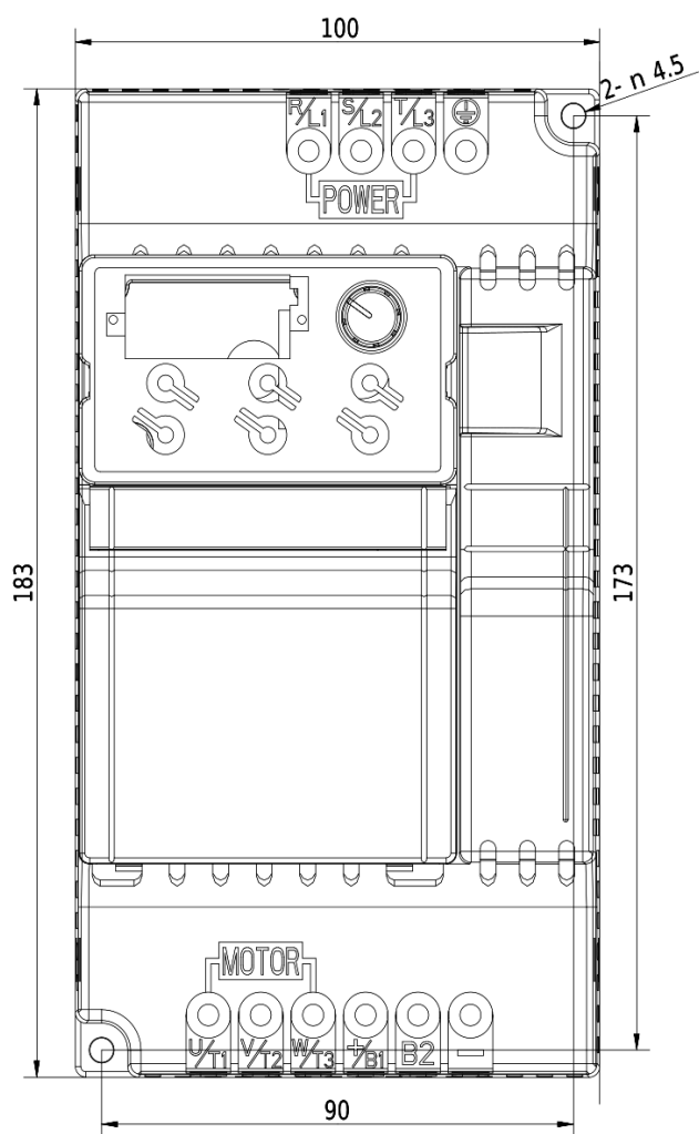
Rozmerový výkres V800 - 2,2kW 2S0022
