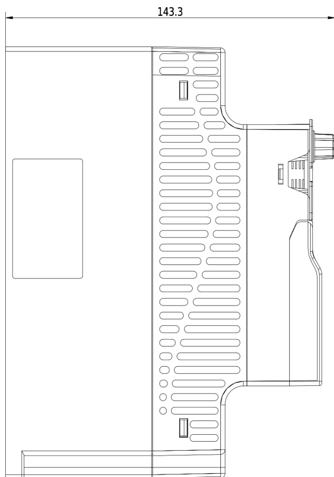
Rozmerový výkres V800 - 2,2kW 2S0022
