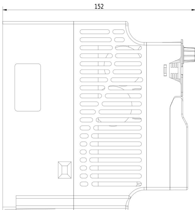
Rozmerový výkres V800 - 0,4kW 2S0004
