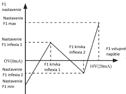
Obrázok 4-29 Schéma krivky 4 a 5
