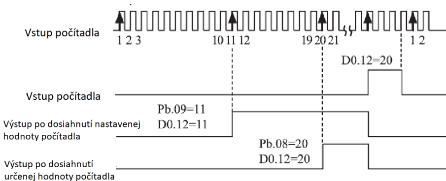
Obrázok 4-27: Dosažená nastavená hodnotu počítadla
