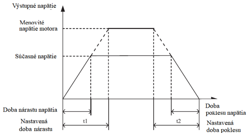
Obrázok 4-7: Priebeh napätia pri V/F separácii
