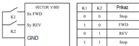
Obrázok 4-8: Nastavenie dvojvodičového režimu 1
