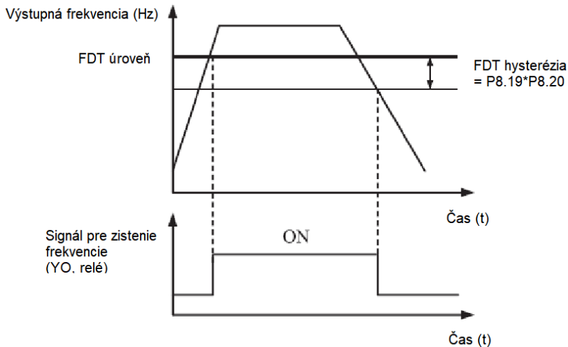
Obrázok 4-14: FDT úrovně
