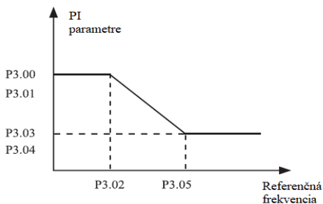
Obrázok 4-4: Vzťah medzi frekvenciou chodu a parametrami PI
