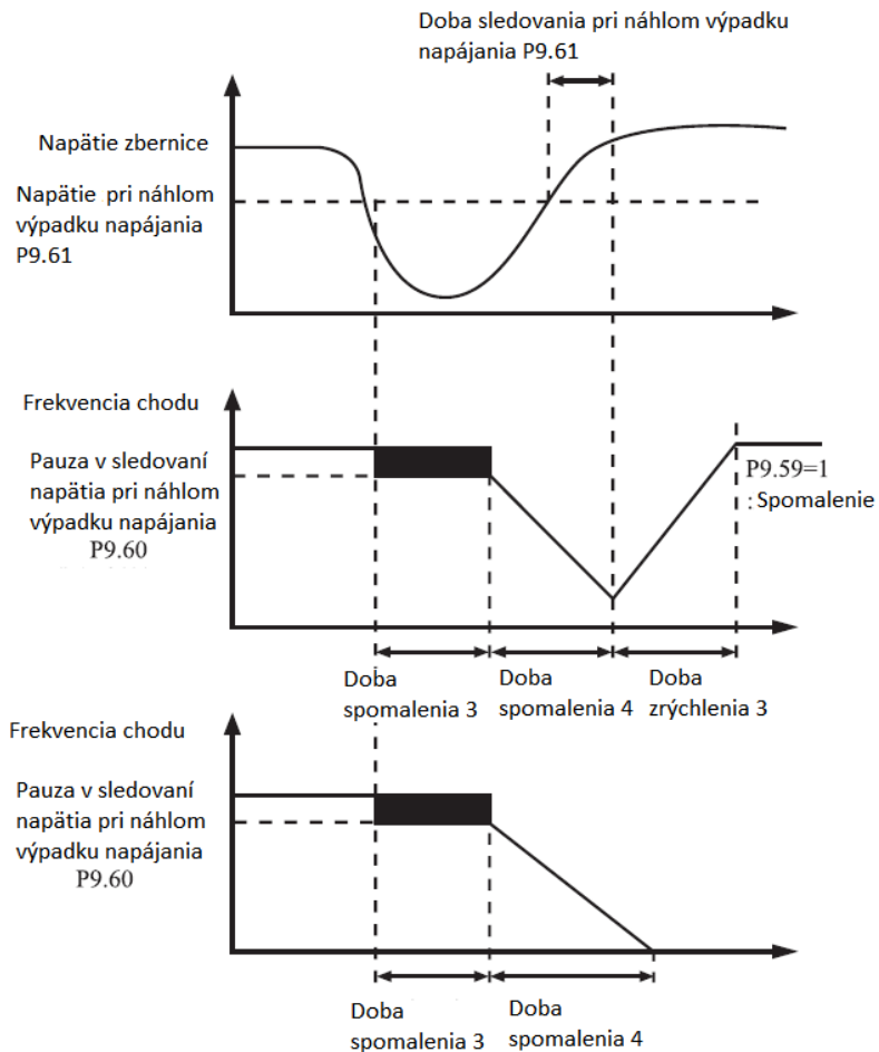
Obrázok 4-22: Činnosť meniča po náhlom výpadku napájania
