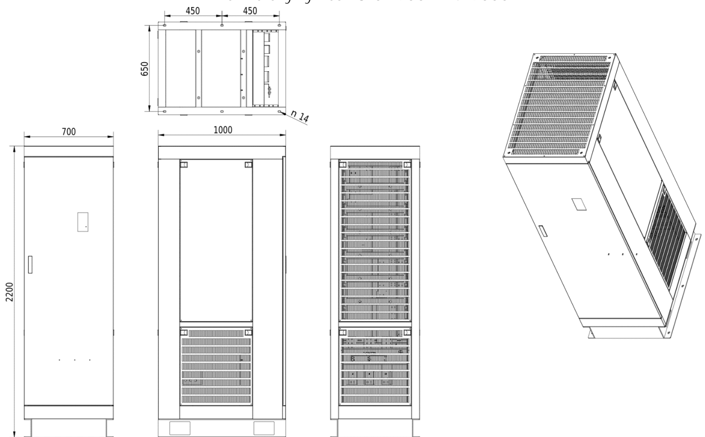
Rozmerový výkres V810 - 900kW 4T9000
