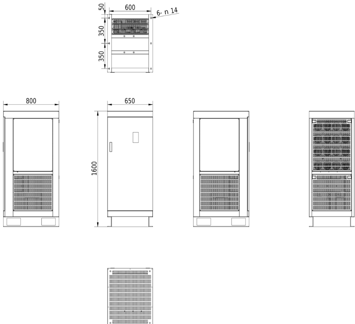
Rozmerový výkres V810 - 630kW 4T6300
