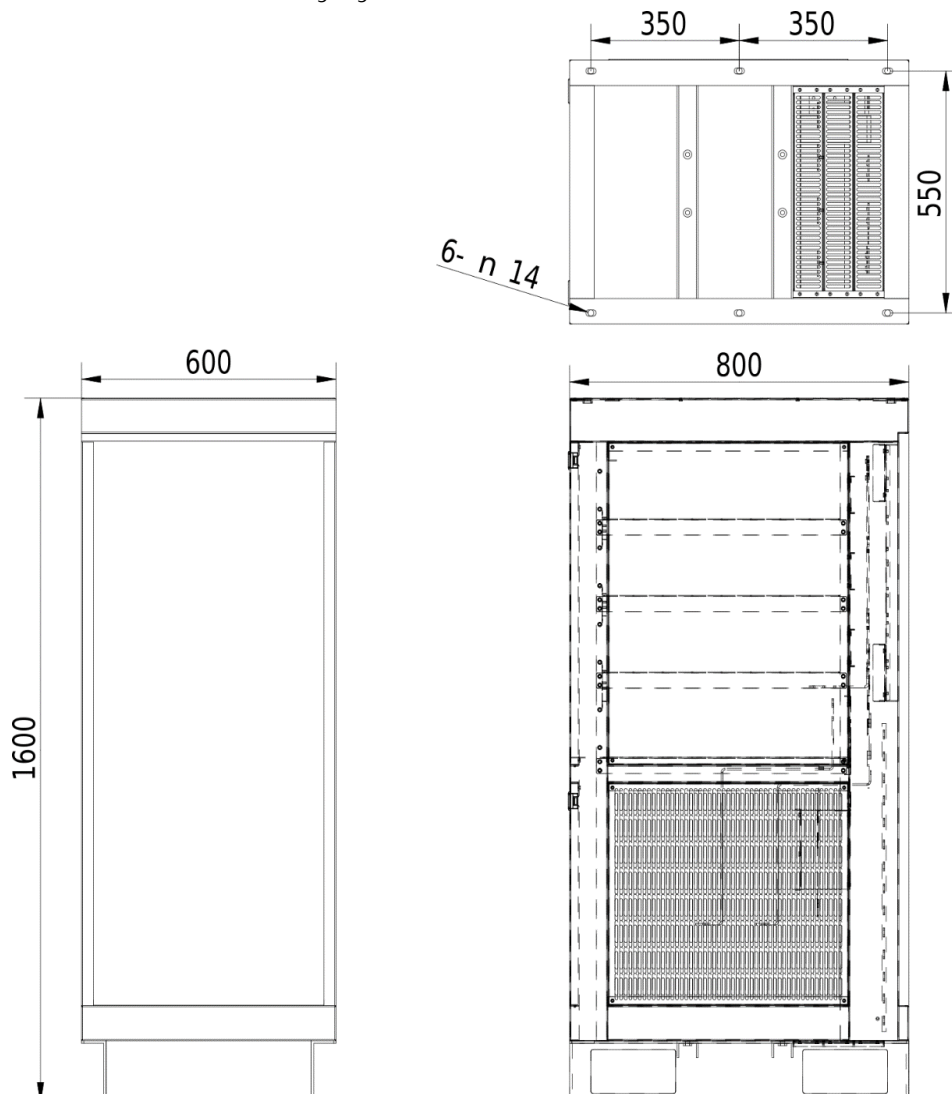
Rozmerový výkres V810 - 450kW 4T4500
