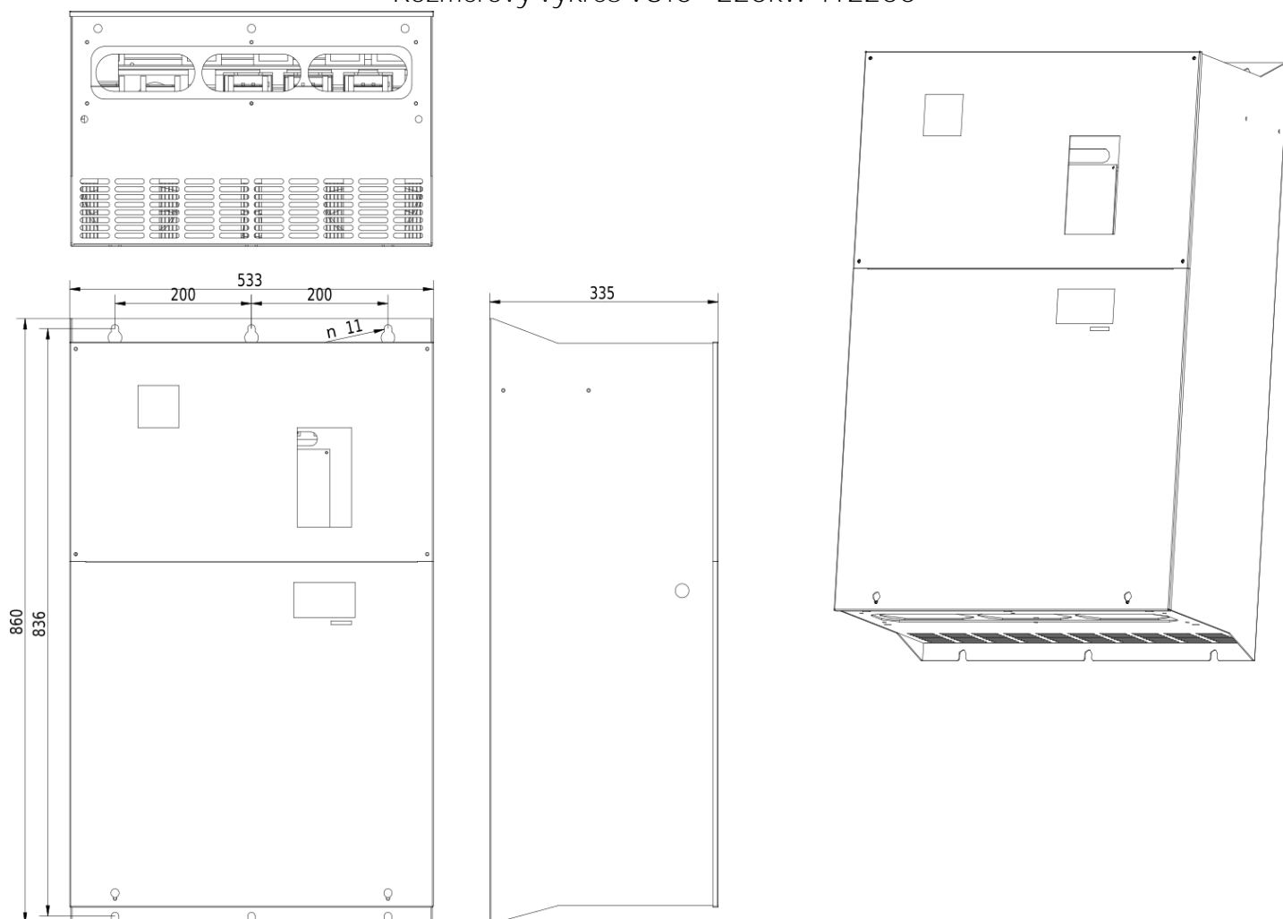
Rozmerový výkres V810 - 220kW 4T2200
