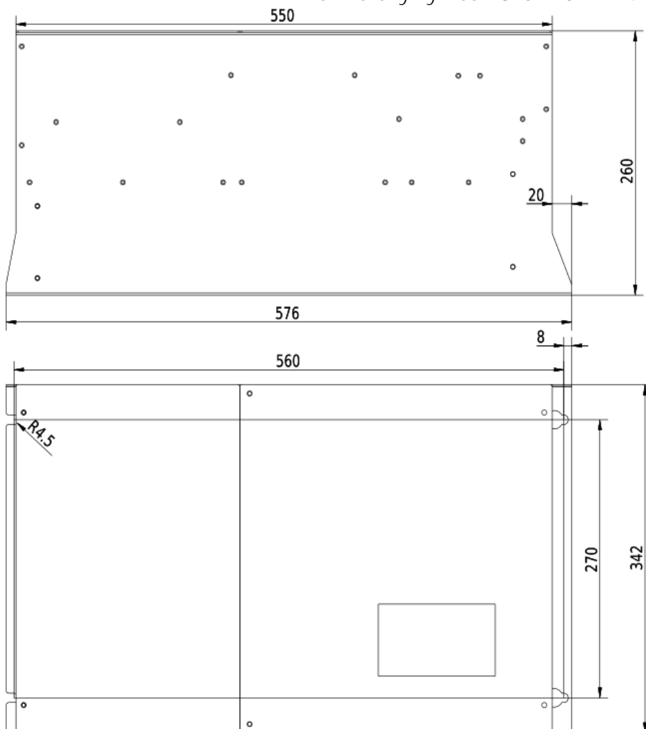
Rozmerový výkres V810 - 132kW 4T1320
