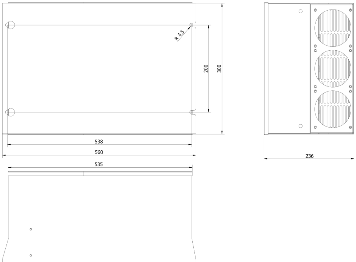
Rozmerový výkres V810 - 75kW 4T0750
