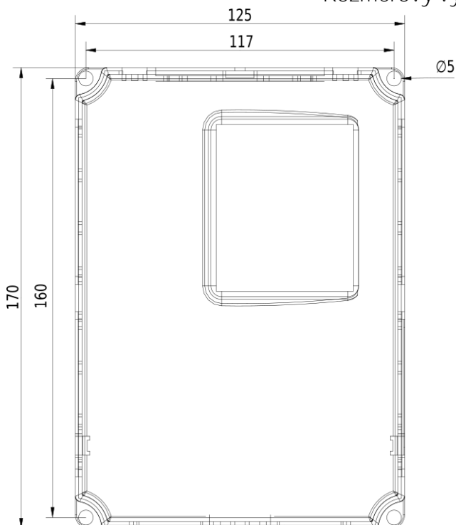
Rozmerový výkres V810 - 1,5kW 4T0015
