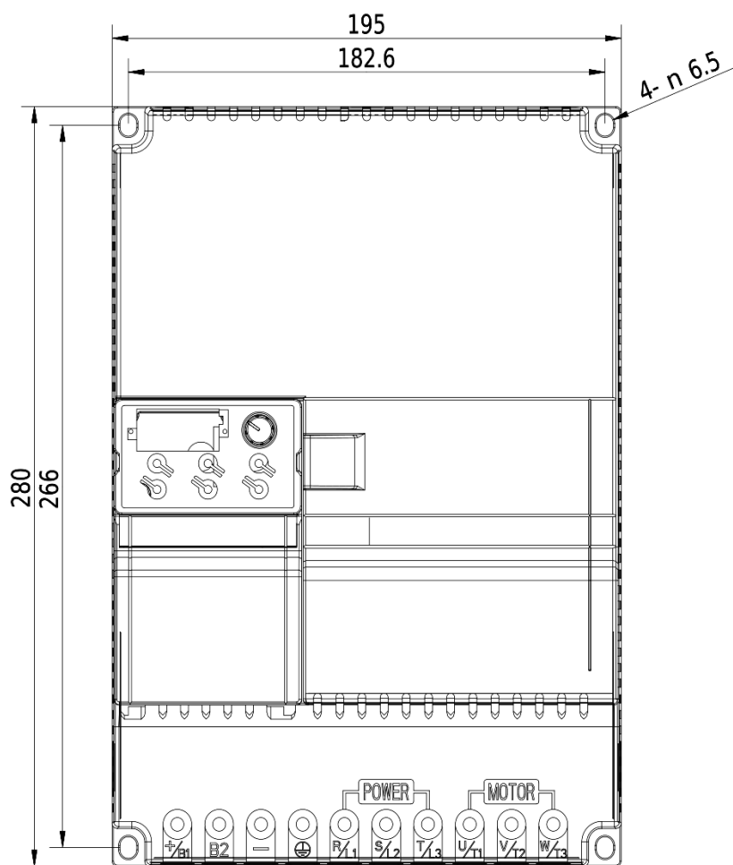
Rozmerový výkres V800 - 22kW 4T0220
