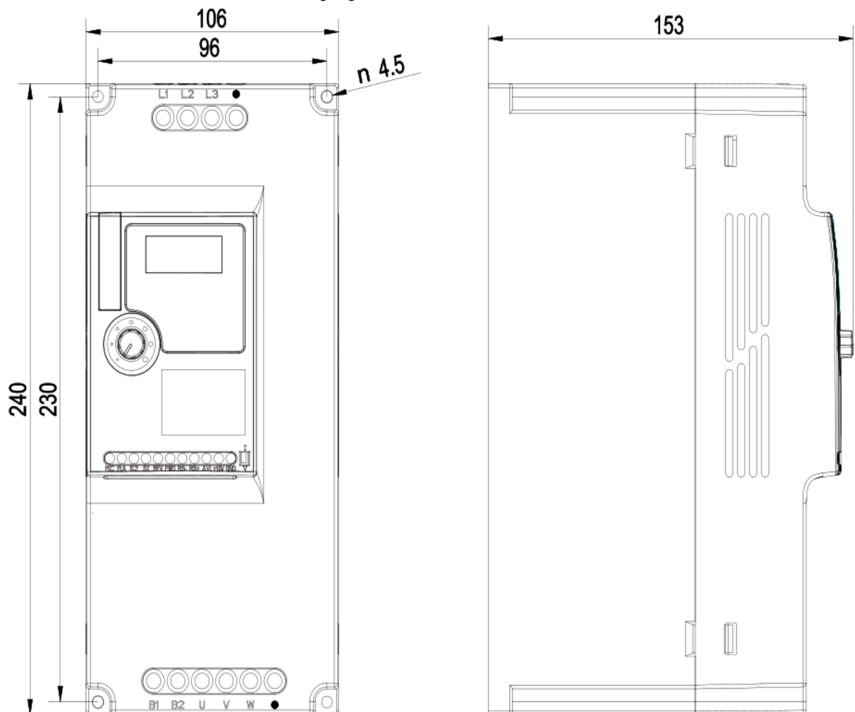
Rozmerový výkres A550 PLUS - 11kW 4T0110
