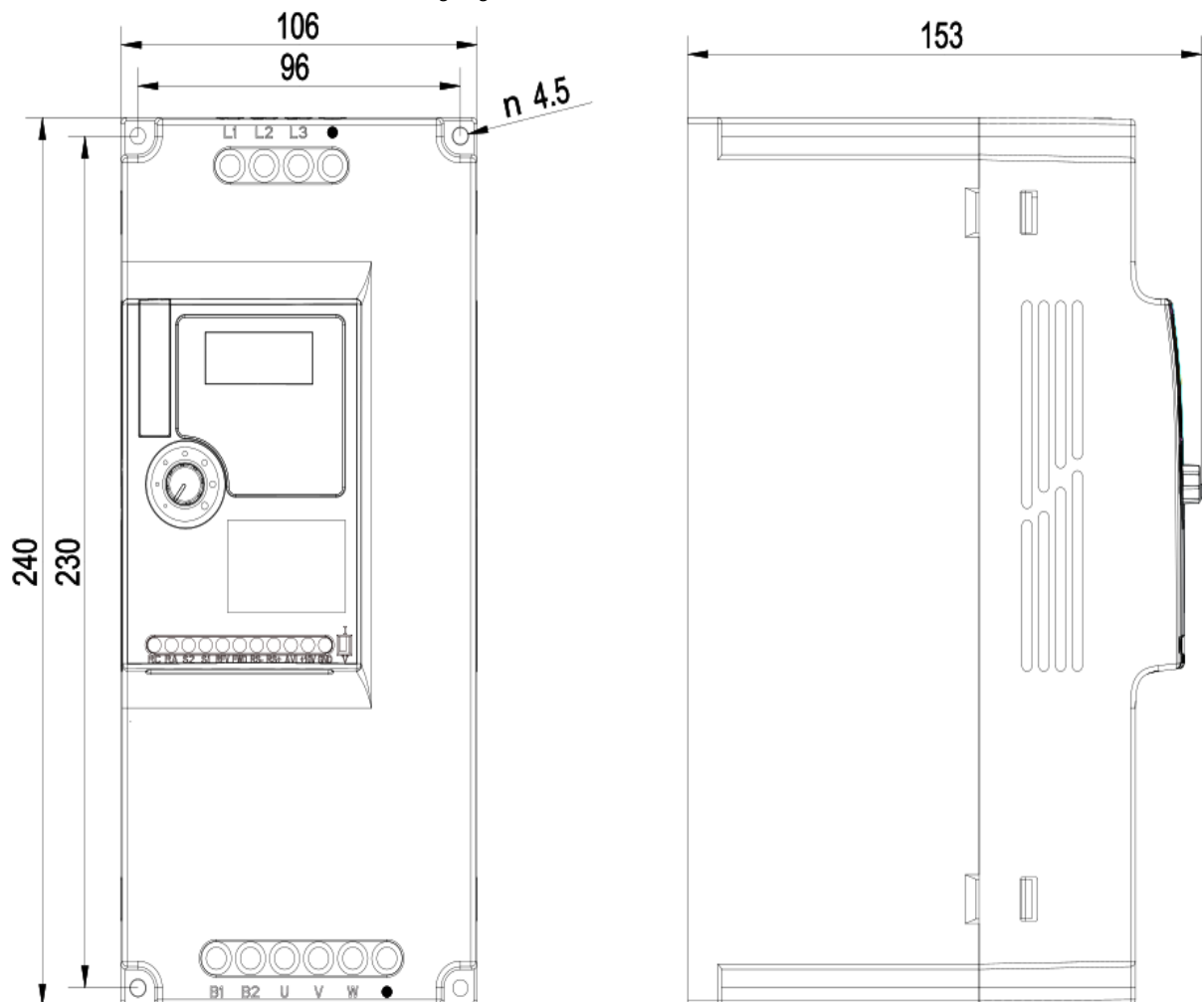
Rozmerový výkres A550 PLUS - 7,5kW 4T0075
